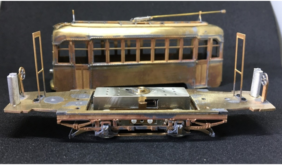
台車廻り
