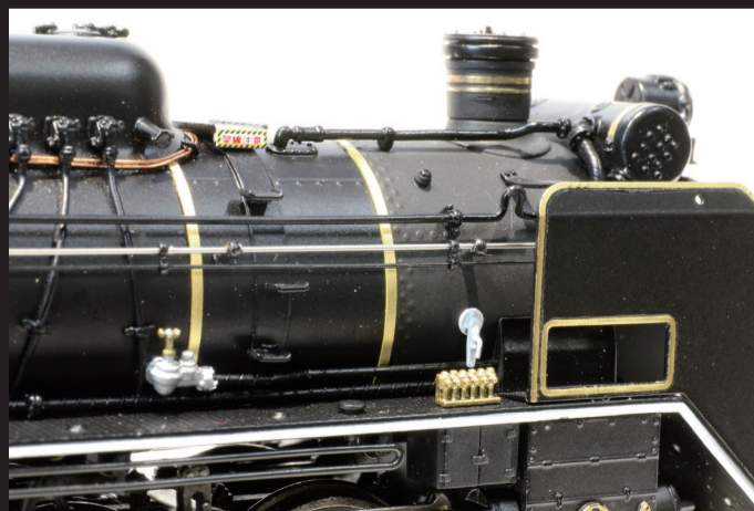
● 1本ずつ独立した空気作用管。ボイラーバンドもエッチングではなく別巻きです。 ● 煙室扉開閉。中には煙管の表現も… —そして、 カンタム・システム搭載
