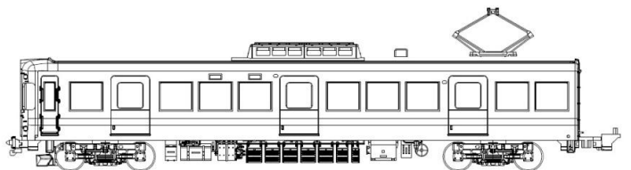
▲パンタ部屋根板切継ぎパーツ、自然通風式抵抗器なども新規製作
